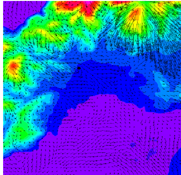
(d) 1200 UTC
